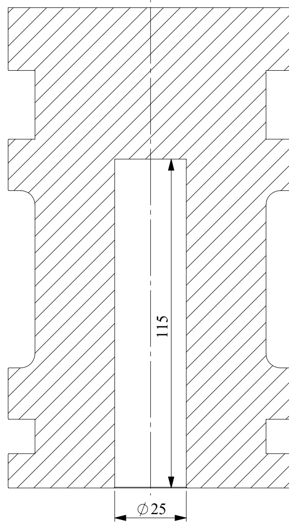
KESIT F-F ÖLÇEK 1 : 1.3
