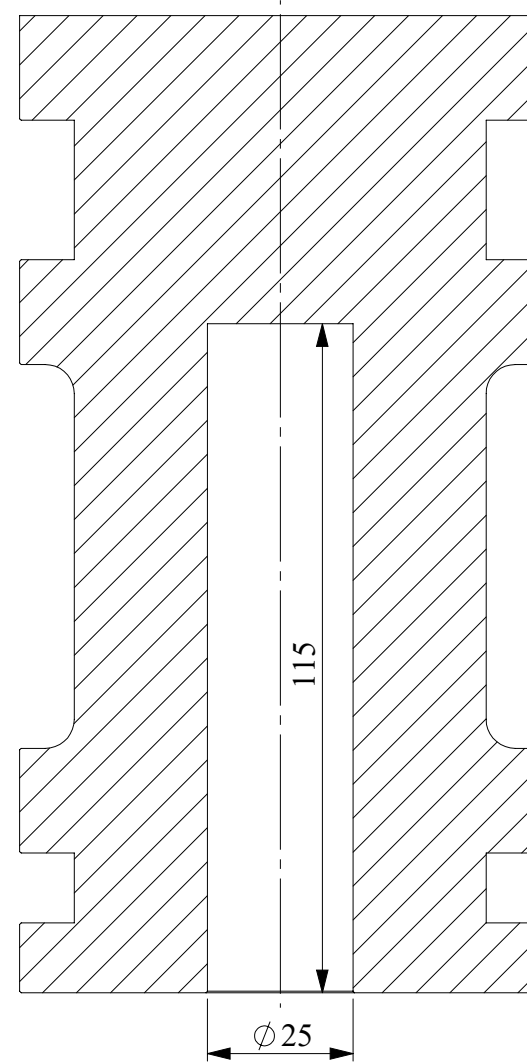
KESİT F-F ÖLÇEK 1 : 1.3
